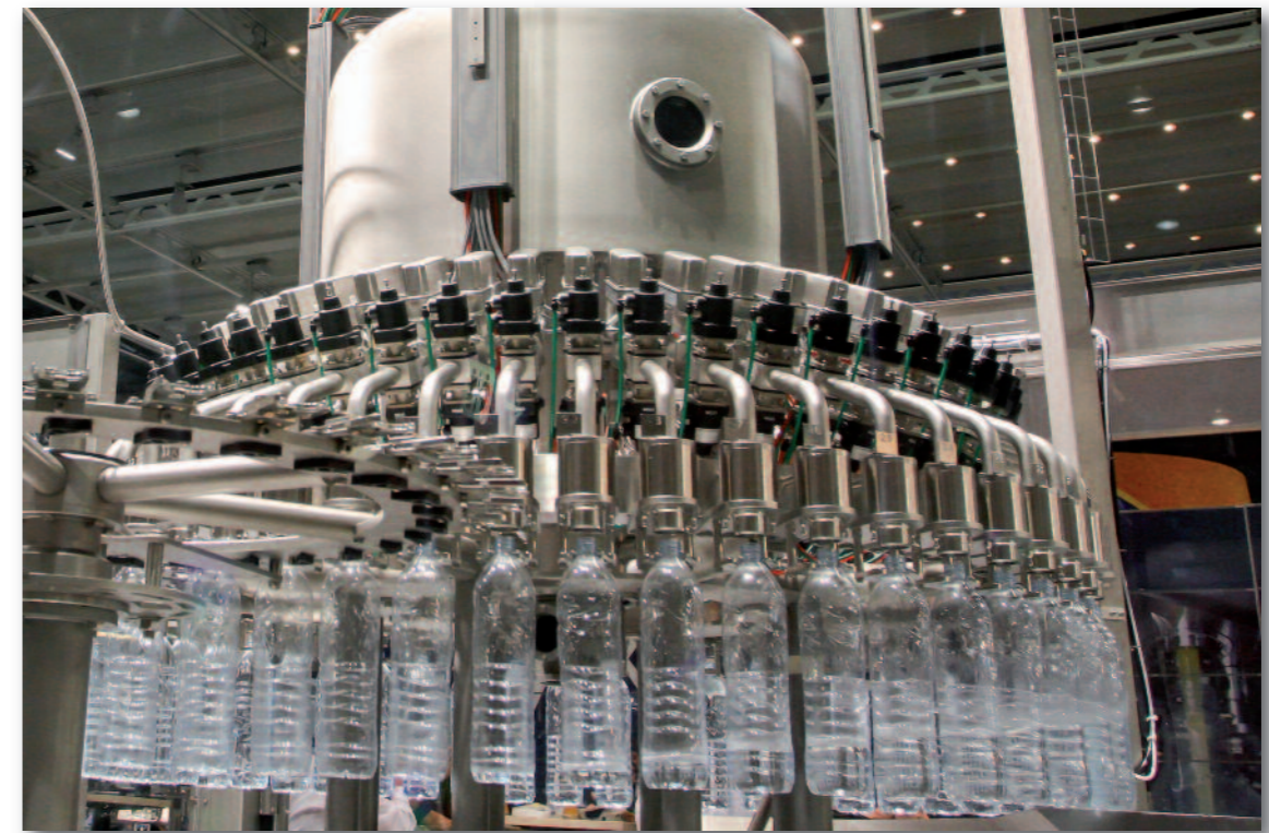
Riempitrice e soffiatrice
