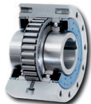
Ruote libere in acciaio inox
